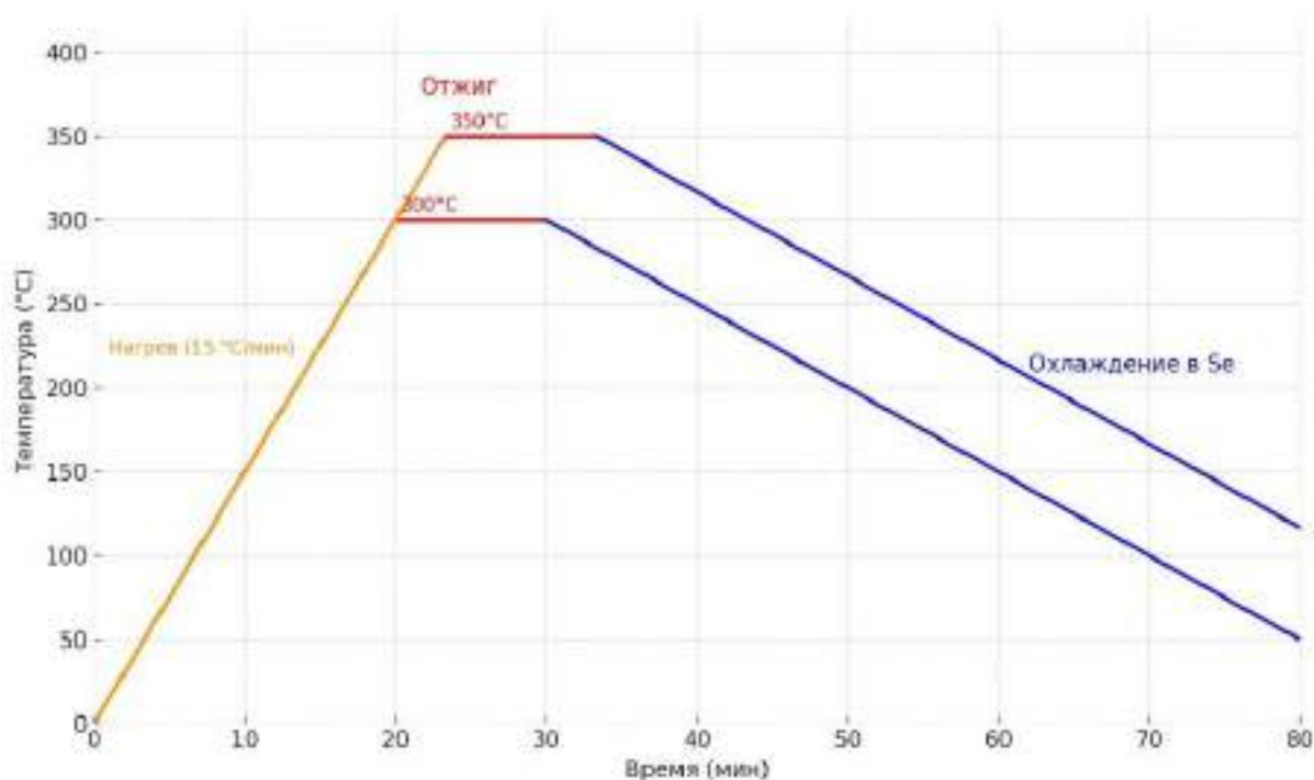
Рисунок 6 - Профили температуры процесса селенизации при двух различных максимальных значениях 300 и 350°C
