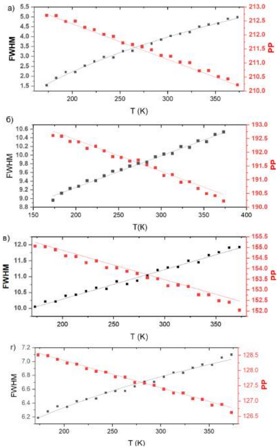
Рисунок 27 – Зависимость положения пиков и их полуширин от температуры измерения
