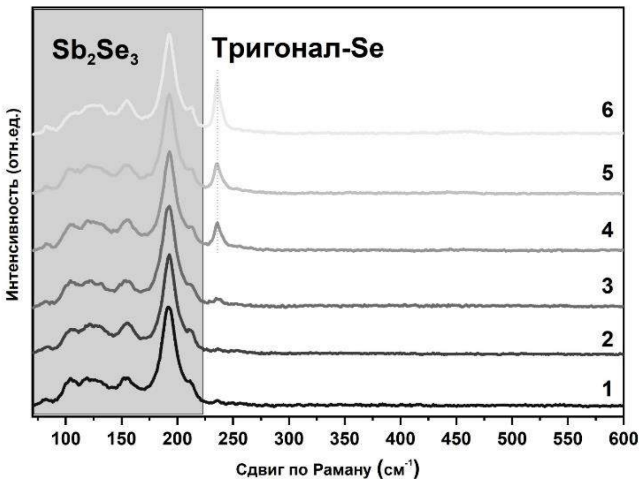
Рисунок 23 – Раман-спектры конкретных участков при определенном подборе лазеров
