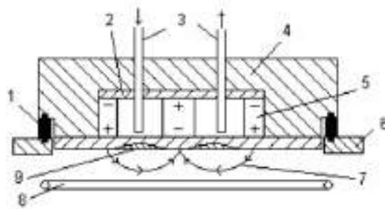
Рисунок В.1 – Конструкция кольцевого магнетрона с водоохлаждением и постоянными магнитами
