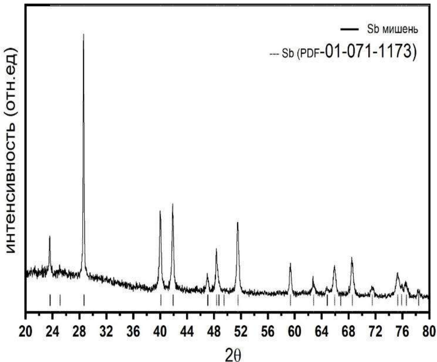
Рисунок 12 – Дифрактограмма мишени Sb
