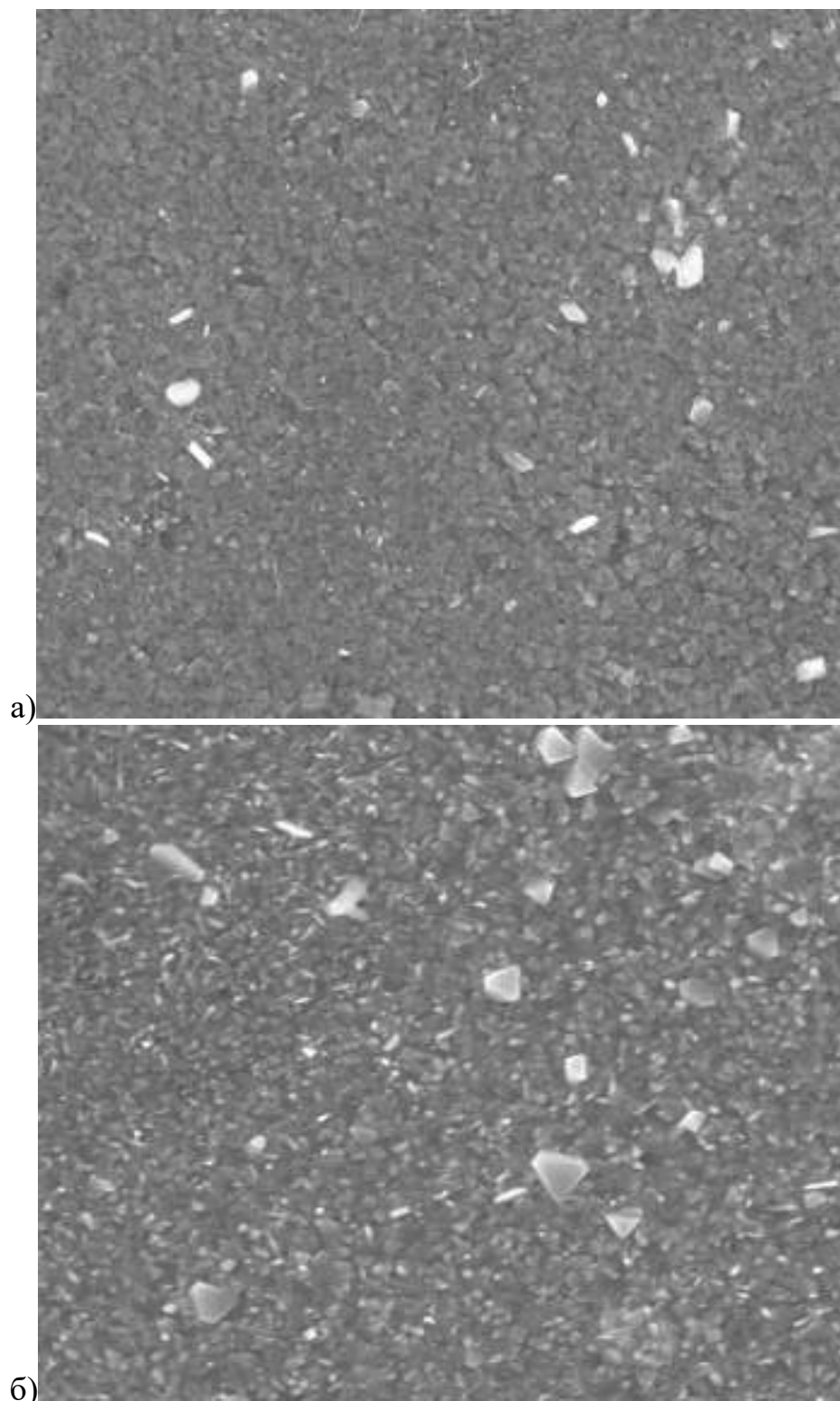
Рисунок 17 – СЭМ изображение плёнок Sb_2Se_3 полученные при режиме 20 кВ, при разрешении X3000, при масштабе 5 мкм при а) 300°C; б) 350°C
