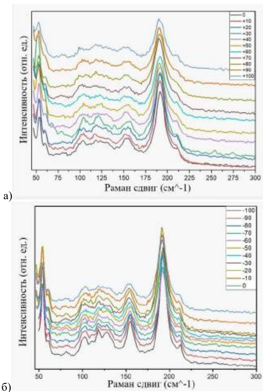
Рисунок 24 – Раман-спектры в диапазоне температур: а) от 0 до +100°С; б) от –100 до 0 °С
