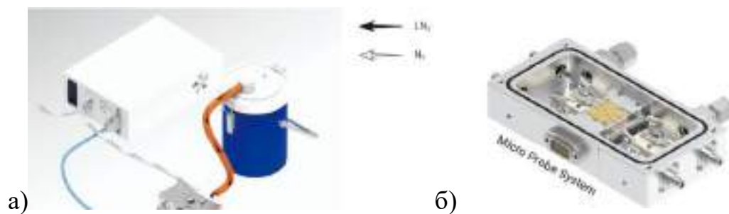
Рисунок 10 – Прибор для нагрева и охлаждения плёнки сконструированная в Университете Авейру, где а) предоставлен сам прибор; б) блок для образца с системой регистрации и подачи температурных измерений с системой нагрева и охлаждения
