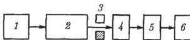
Блок-схема спектрофотометра:
