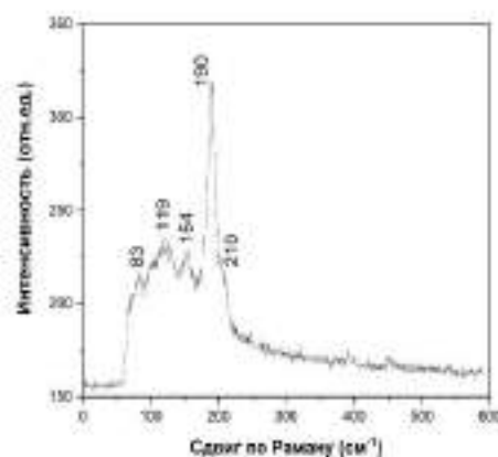
Рисунок 21 – Раман-спектры образцов плёнок Sb_2Se_3 при а) 300°С; б) 350°С
