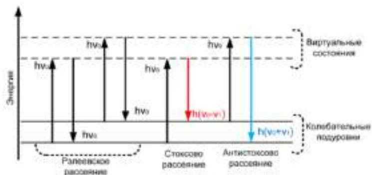
Рисунок Б.1 – Схема регистрации КР-спектров
