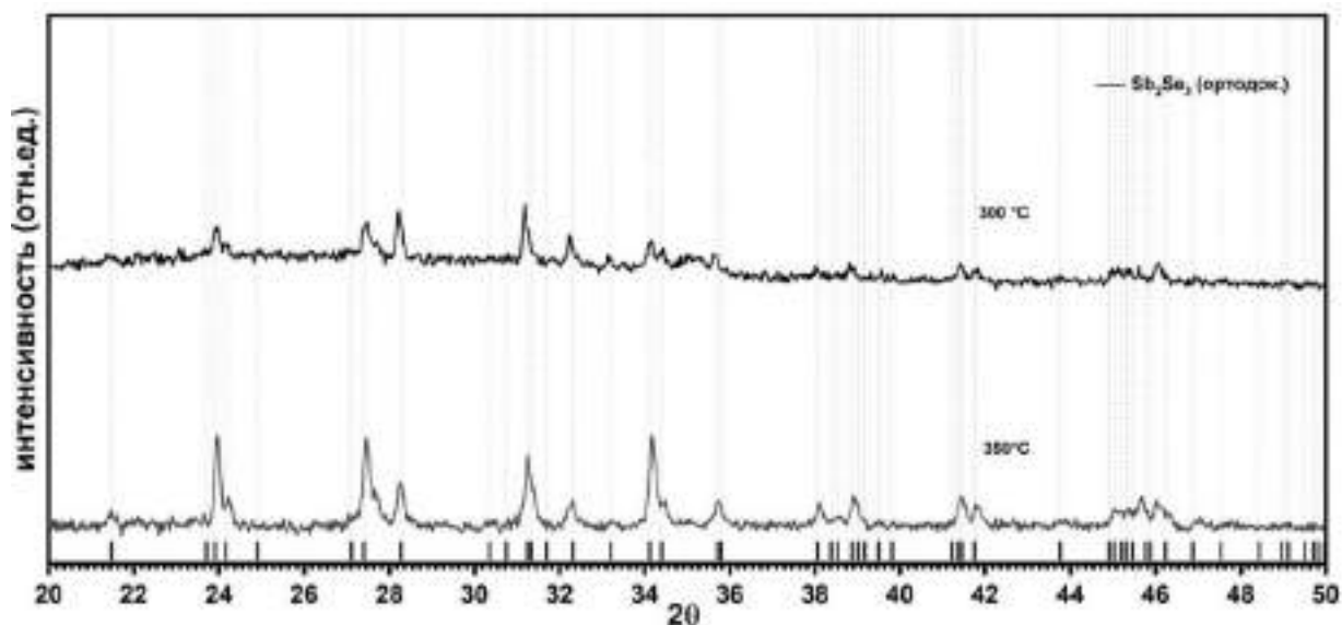
Рисунок 19 – Дифрактограмма образцов плёнок Sb 2 Se 3 при 300°C и 350°C
