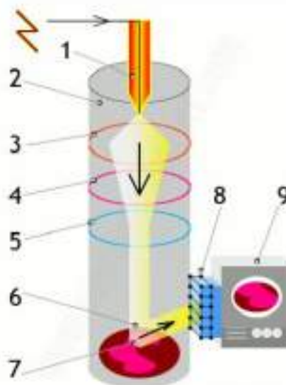
Рисунок Г.2 - Принципиальная схема SEM: 1- электронная пушка; 2- вакуумная камера; 3- анод; 4,5 – электромагнитные катушки; 6- электронный луч; 7 – обратные электроны; 8- детектор; 9- экран для вывода изображения
