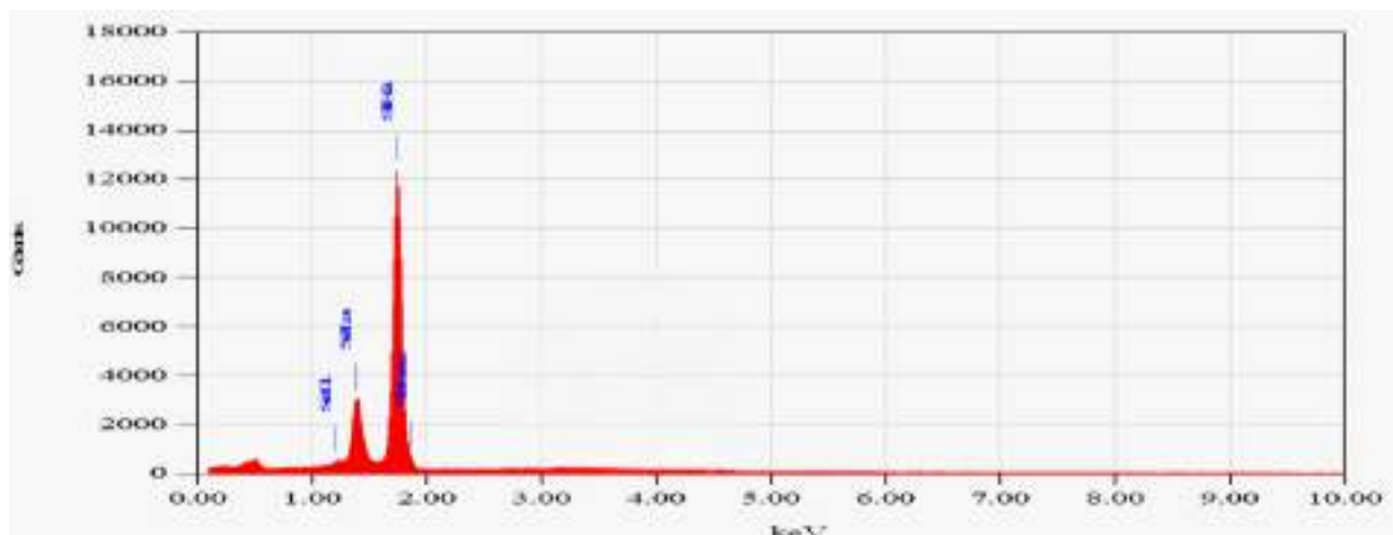
Рисунок Ё.1 – ЭДС – анализ для пленки селенида сурьмы, полученных селенизацией пленки сурьмы, осажденных магнетронным методом
