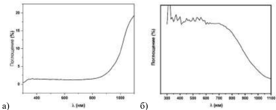
Рисунок 19 – Спектры поглощения плёнок Sb_2Se_3 при а) 350°C; б) 300°C
