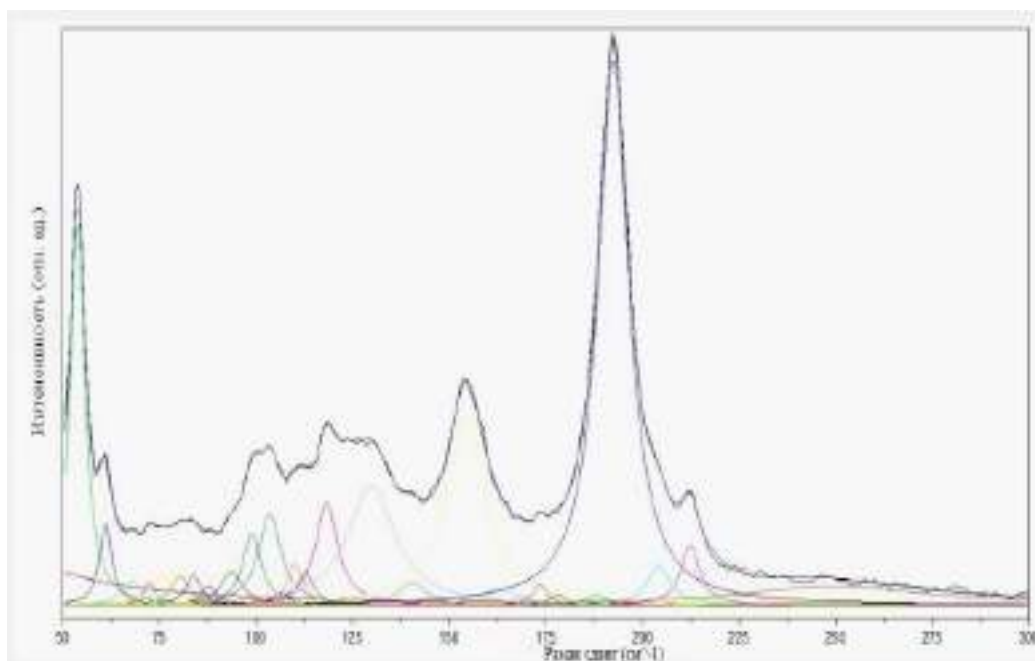
Рисунок 25 – Аппроксимация кривой спектра, полученного при температуре 0 °С функцией Войта полученная программой Origins
