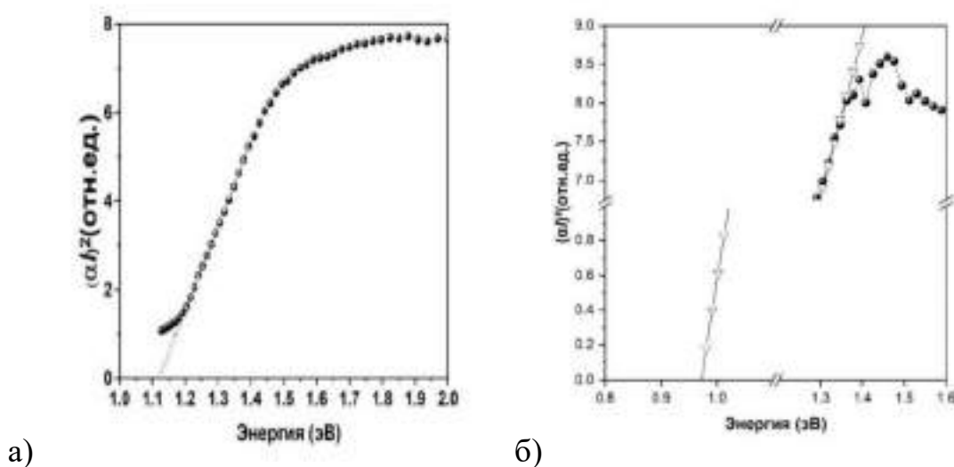
Рисунок 20 – Спектры пропускания плёнок Sb_2Se_3 при а) 350°C; б) 300°C
