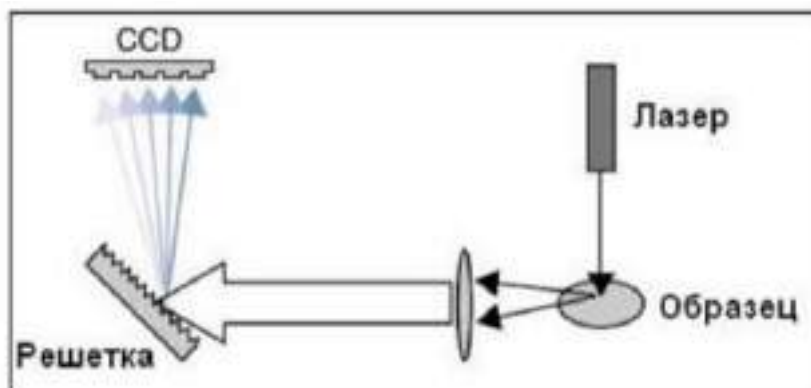
Рисунок Б.1 – Схема регистрации КР-спектров
