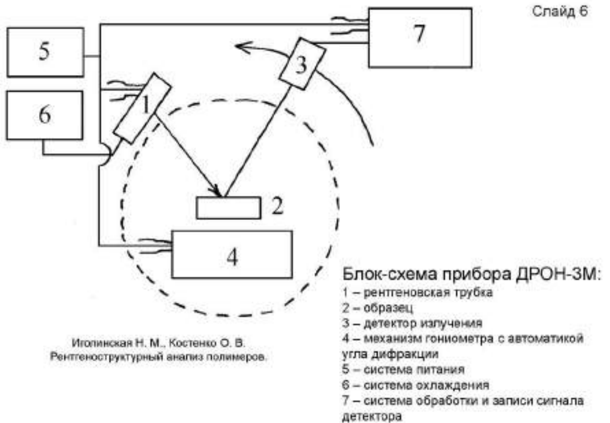
Рисунок Д.2 – Схема рентгеноструктурного устройства в Физико-техническом университете
