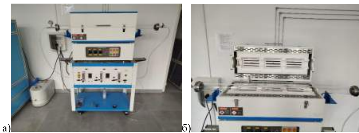
Рисунок 3 – CVD установка, где а) Сам аппарат; б) Внутренняя часть куда помещались порошок Se и подложки Sb (сама схема фотографии изображена на рисунке 5)
