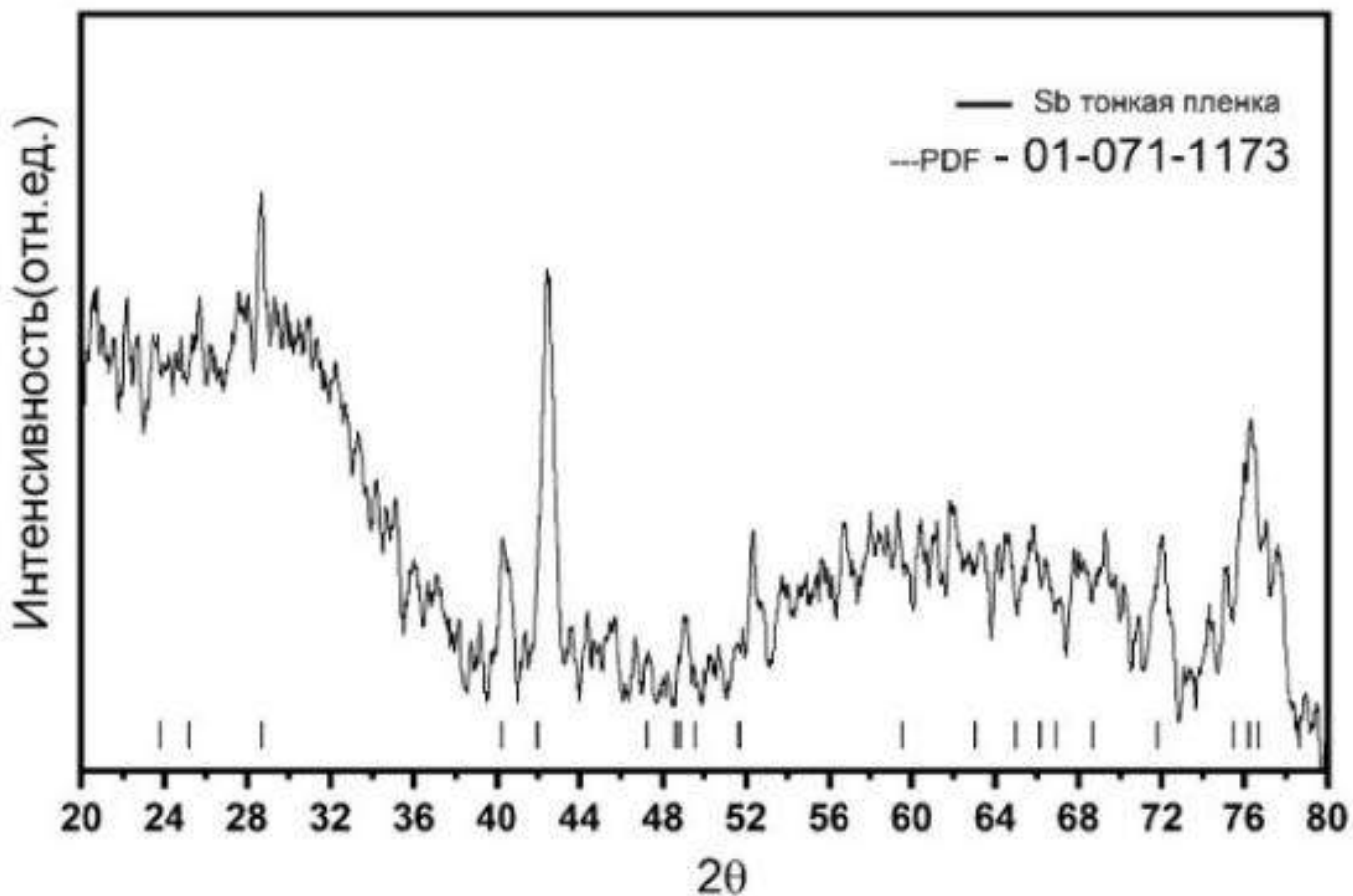
Рисунок 14 - Дифрактограмма плёнки Sb
