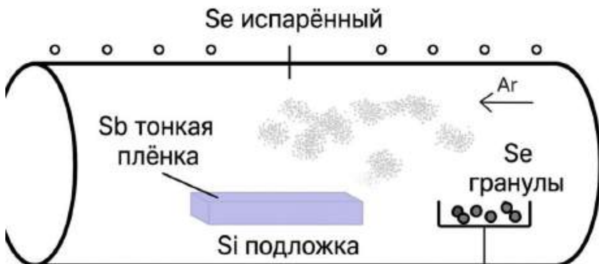
Рисунок 5 – Процесс селенизации в CVD-установке
