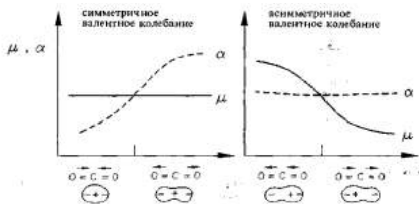
Рисунок Б.3 - Изменение поляризуемости и дипольного момента в ходе колебаний молекулы CO 2
