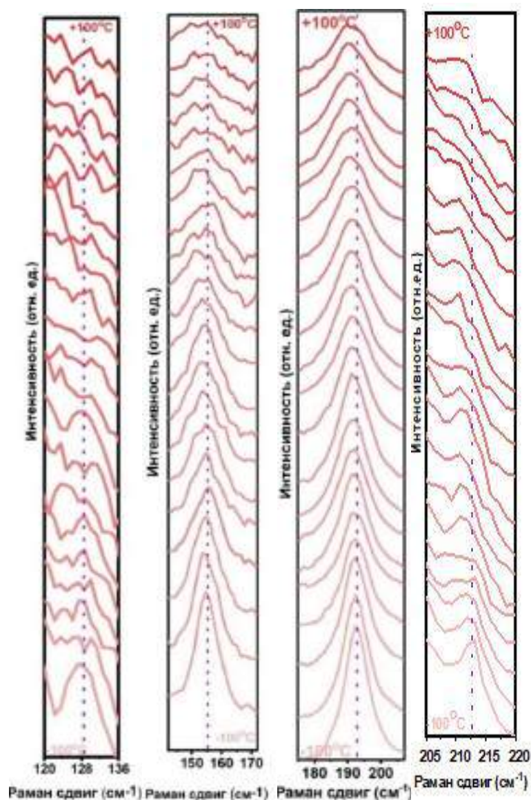
Рисунок 26 – Пики аппроксимационных кривых спектров наиболее интенсивных линий по рисунку 25 полученных программой Origin
