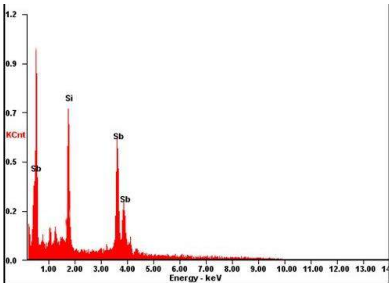
Рисунок 13 – ЭДС-анализа плёнки Sb
